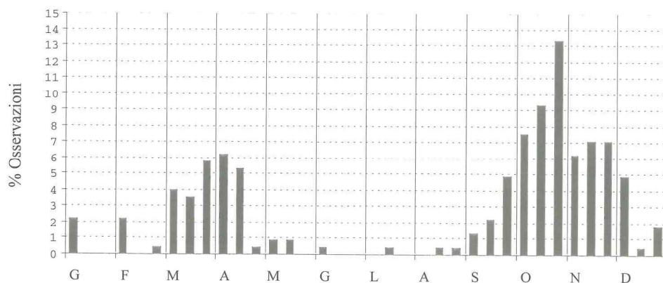
Fig. 1. fenologia stagionale del Gufo di palude in Italia per decenni.
